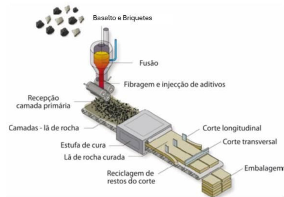
Figura 2: Representa esquematicamente o processo produtivo da lã de rocha.
