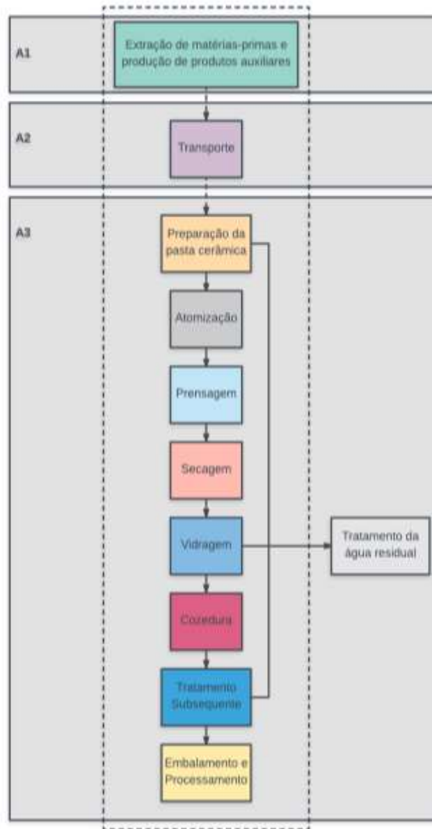
Figura 1 - Etapas da produção do grés porcelânico (A1-A3).
